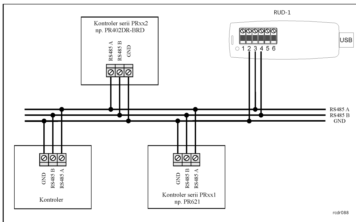
Rys. 1 Schemat podłączenia interfejsu RUD-1 do systemu kontroli dostępu RACS4
