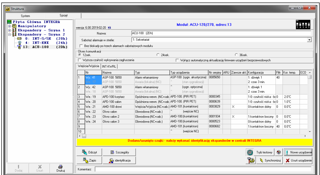
Rys. 19. Program DLOADX: informacje wyświetlane po zarejestrowaniu nowego urządzenia w kontrolerze połączonym do centrali INTEGRA / INTEGRA Plus.
