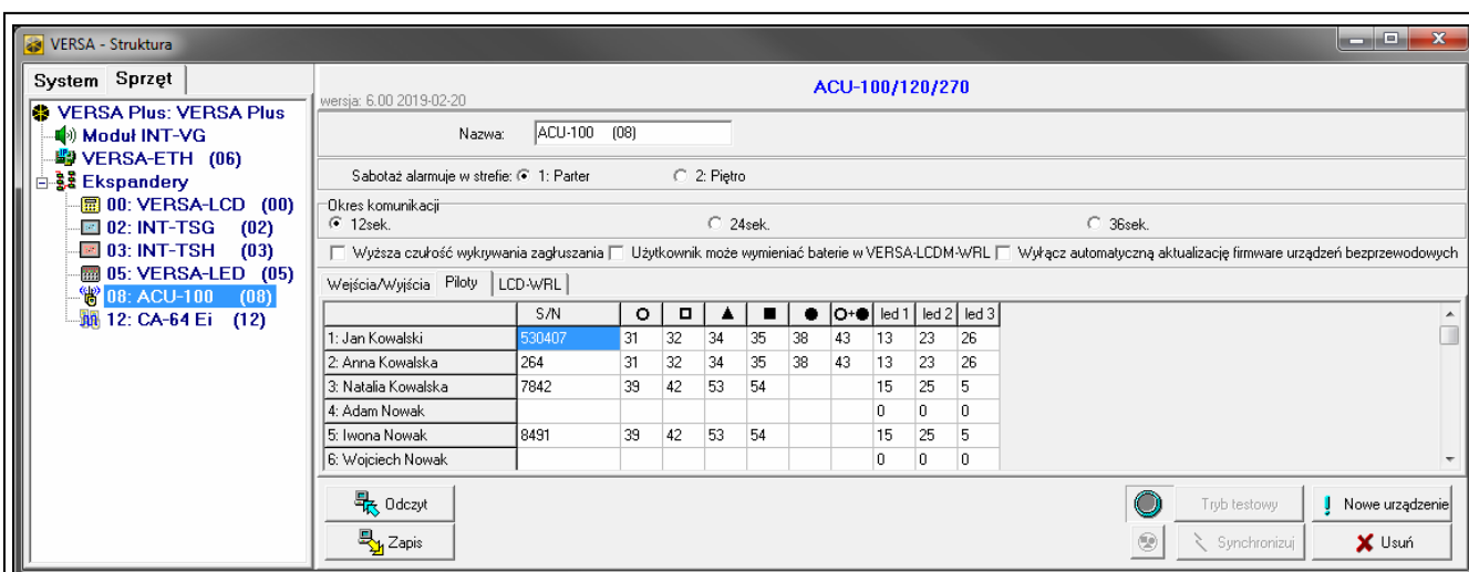
Rys. 23. Program DLOADX: zarządzanie pilotami w przypadku kontrolera podłączonego do centrali VERSA / VERSA Plus / VERSA IP.
