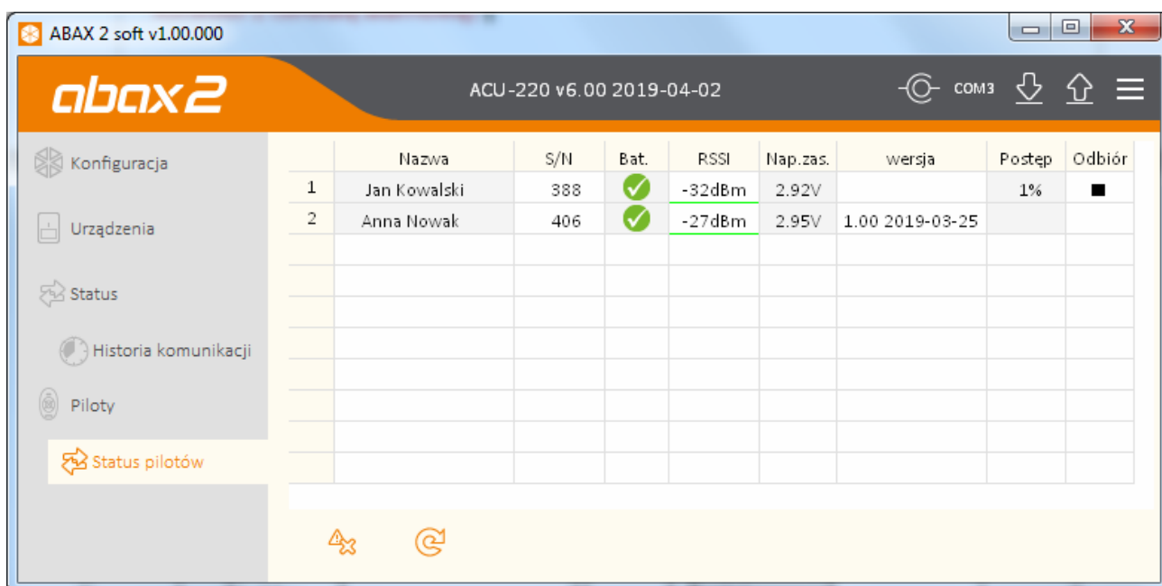
Rys. 17. Program ABAX 2 Soft: zakładka „Status pilotów”.
