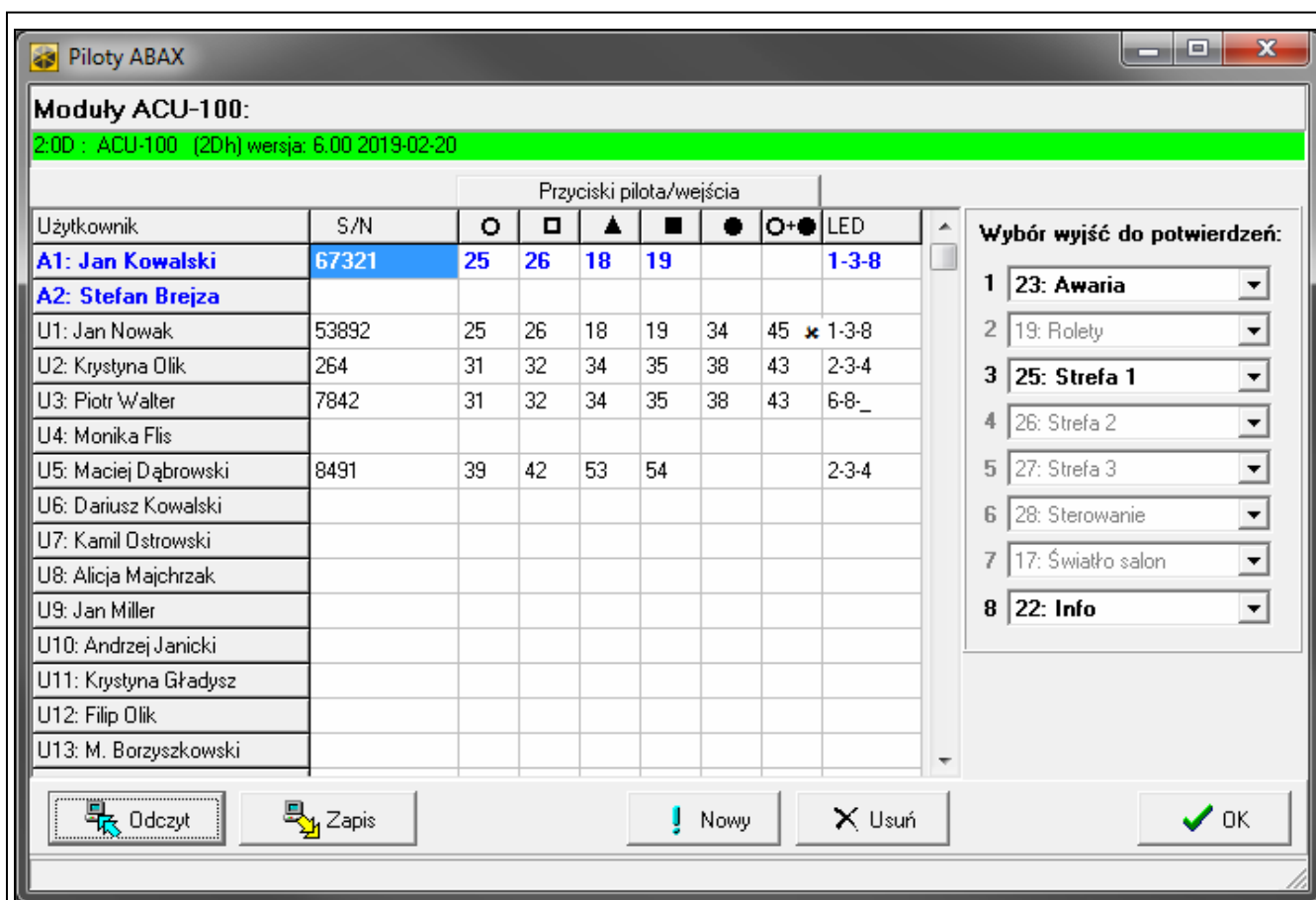
Rys. 22. Program DLOADX: zarządzanie pilotami w przypadku kontrolera podłączonego do centrali INTEGRA / INTEGRA Plus.
