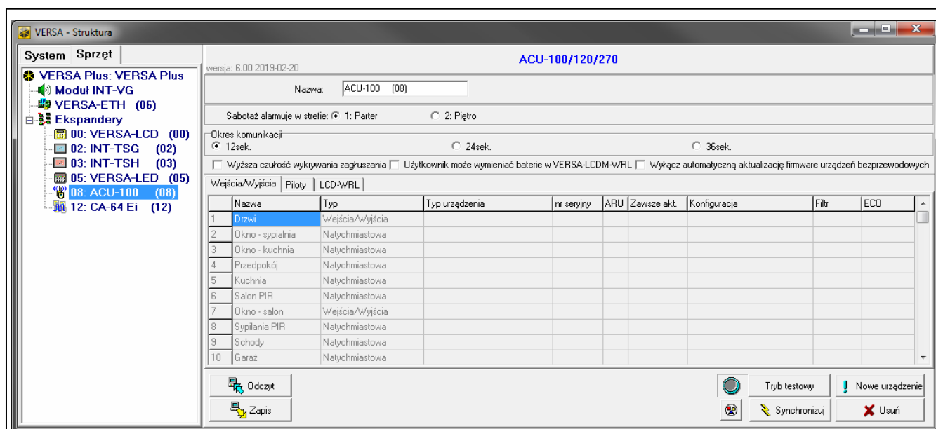
Rys. 21. Program DLOADX: parametry i opcje kontrolera podłączonego do centrali VERSA / VERSA Plus / VERSA IP.
