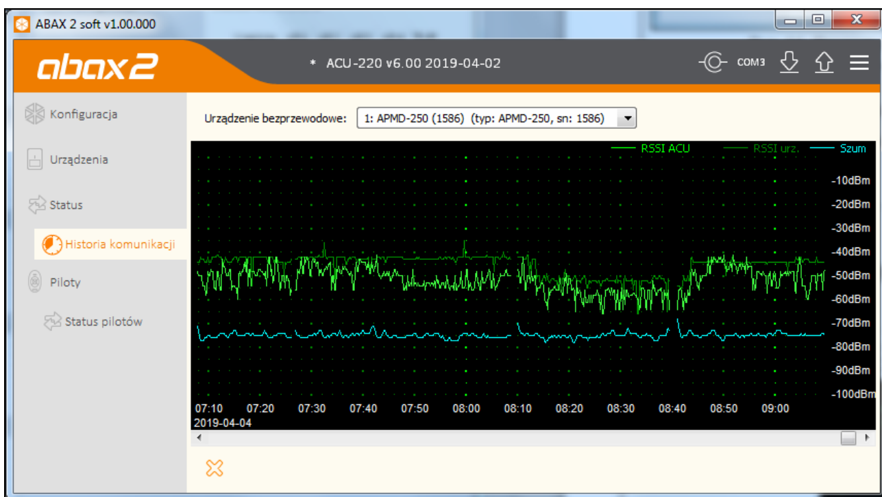
Rys. 14. Program ABAX 2 Soft: zakładka „Historia komunikacji”.
