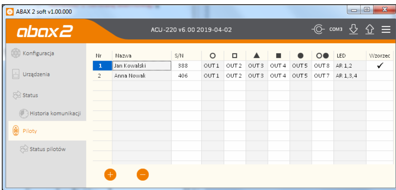
Rys. 16. Program ABAX 2 Soft: zakładka „Piloty”.
