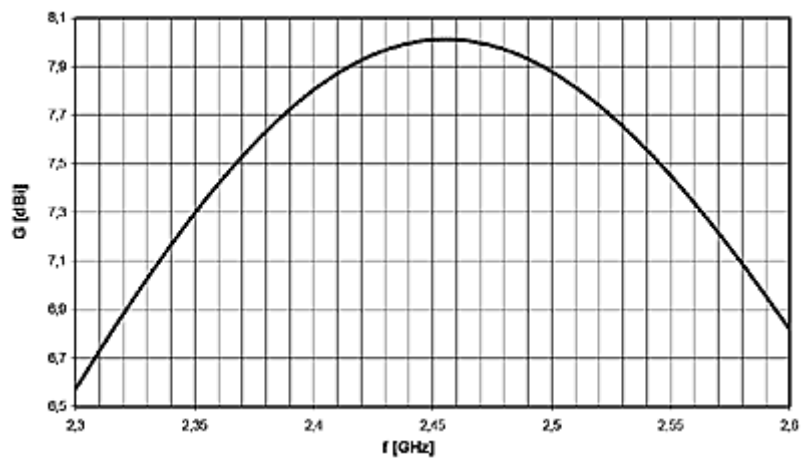
Charakterystyka zysku anteny w funkcji częstotliwości
