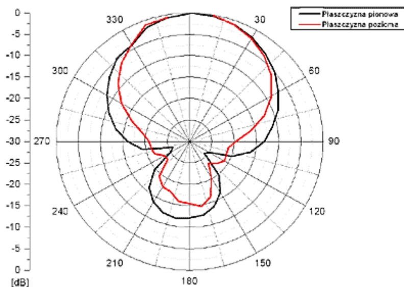
Charakterystyka promieniowania w płaszczyźnie pionowej i poziomej
