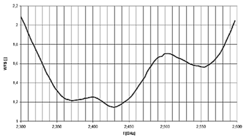
Charakterystyka współczynnika fali stojącej w funkcji częstotliwości
