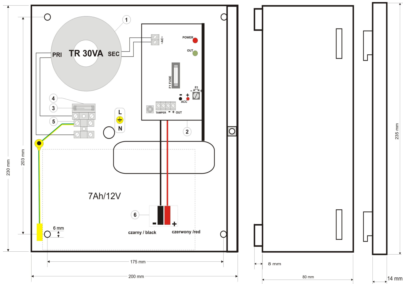
Rys.3. Widok zasilacza.
