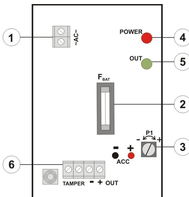
Rys. 2. Widok płyty pcb zasilacza.
