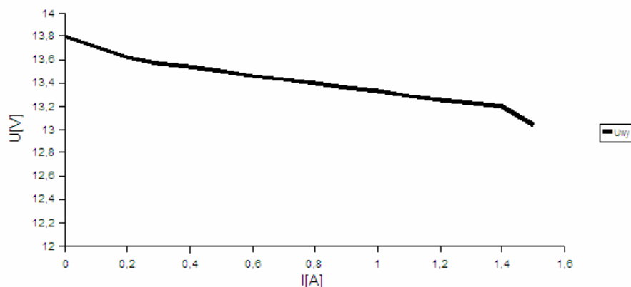
Wykres Uwy(Io)
