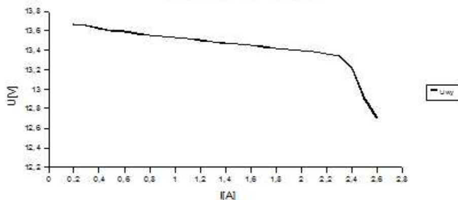
Diagramme Uwy(Io)
