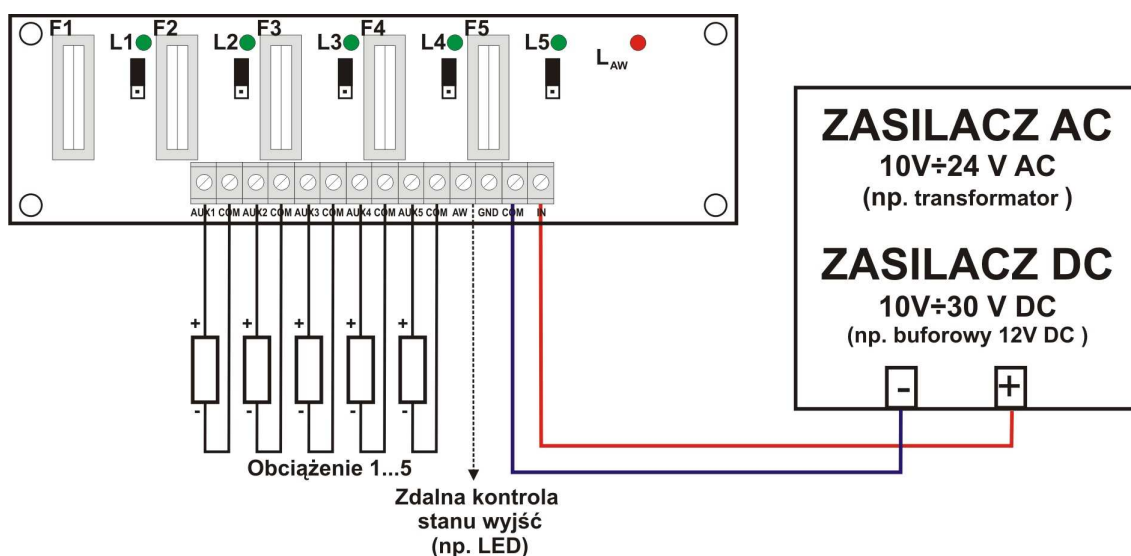
Rys.1. Schemat podłączenia modułu LB5/AW (przykładowy).
