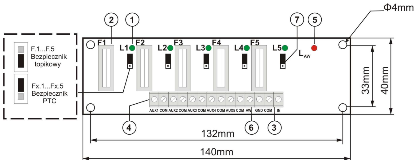
Rys.2. Widok modułu LB5/AW.
