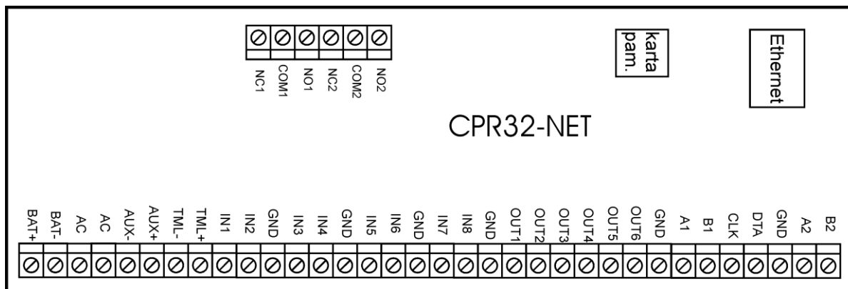
Rys. 1 Centrala CPR32-NET
