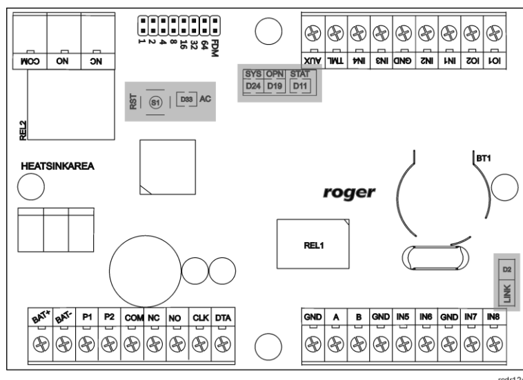
Rys. 3 Wskaźniki LED na płycie centrali CPR32-SE v3.0
