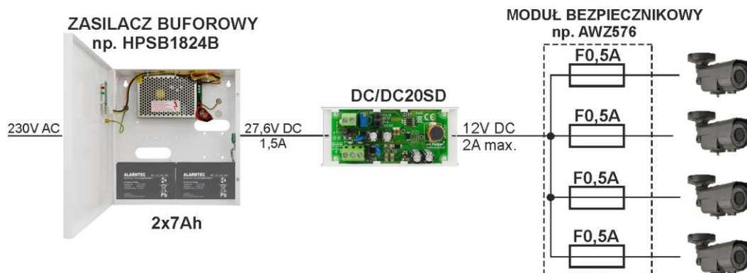
Schemat poglądowy zastosowania przetwornicy.
