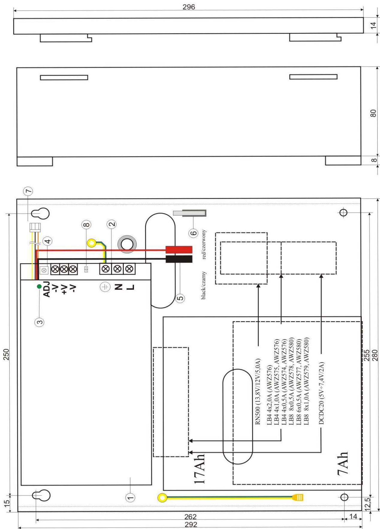
Rys.2. Widok zasilacza.
