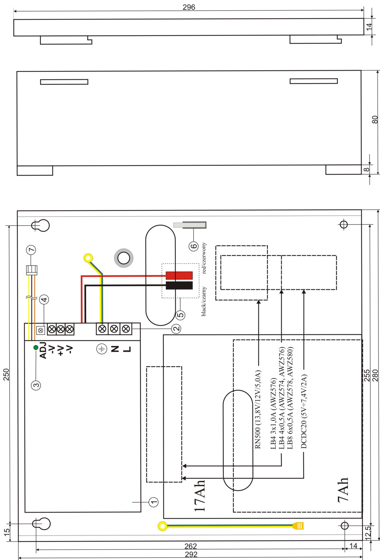
Rys.2. Widok zasilacza.
