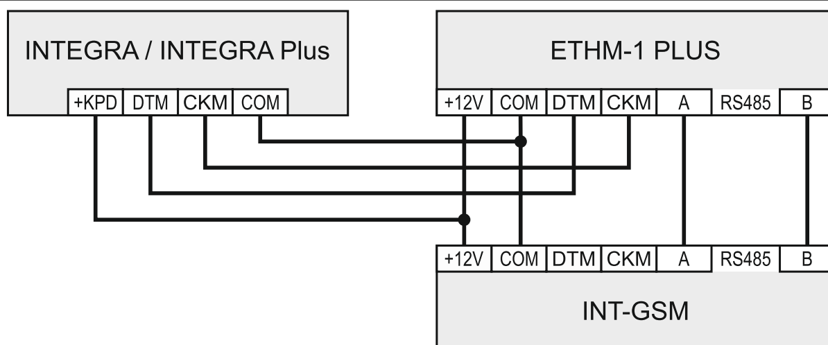
Rys. 7. Sposób podłączenia modułu INT-GSM do modułu ETHM-1 Plus.
