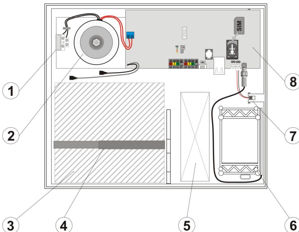
Rys .4 Obudowa centrali sterującej: 1) zaciski zasilania z bezpiecznikiem; 2) transformator zasilania; 3) miejsce na akumulator; 4) obejmująca mocująca akumulator; 5) miejsce na kable; 6) antena GSM; 7) styk przeciw sabotażowy; 8) płyta główna panelu sterowania.
