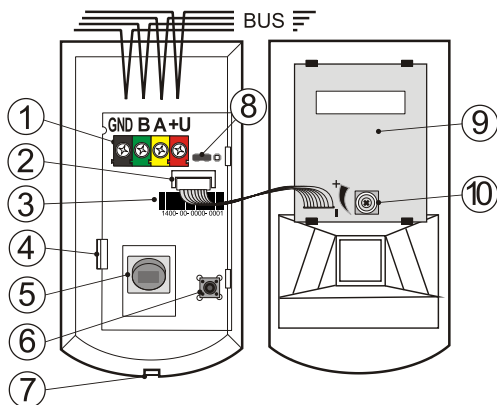
Rysunek: 1 – zaciski magistrali cyfrowej; 2 – wtyczka do podłączenia części MW; 3 – kod produktu; 4 – zatrzask PCB; 5 – sensor PIR; 6 – styk sabotażowy; 7 – zatrzask obudowy; 8 – zworka testu; 9 – sensor MW; 10 – poziom czułości MW;
