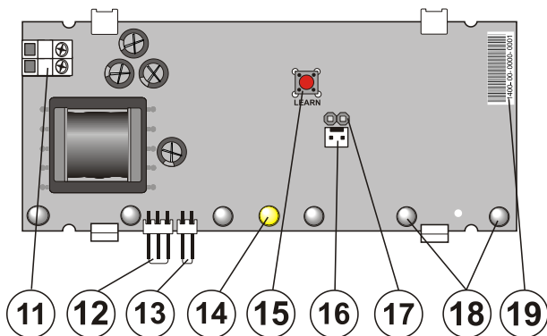
Rysunek: 11 – złącze zasilania 12V DC; 12 – podłączenie syren piezo (uwaga: wysokie napięcie); 13 – podłączenie akumulatora; 14 – żółta dioda wskazująca błąd; 15 – przycisk logowania; 16 – podłączenie zewnętrznej anteny; 17 – zworka zewnętrznej anteny; 18 – alarmowe diody LED; 19 – kod produktu;
