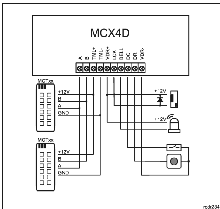
Rys. 5 Typowy scenariusz obsługi przejścia dwustronnego z czynnikiem MCT
