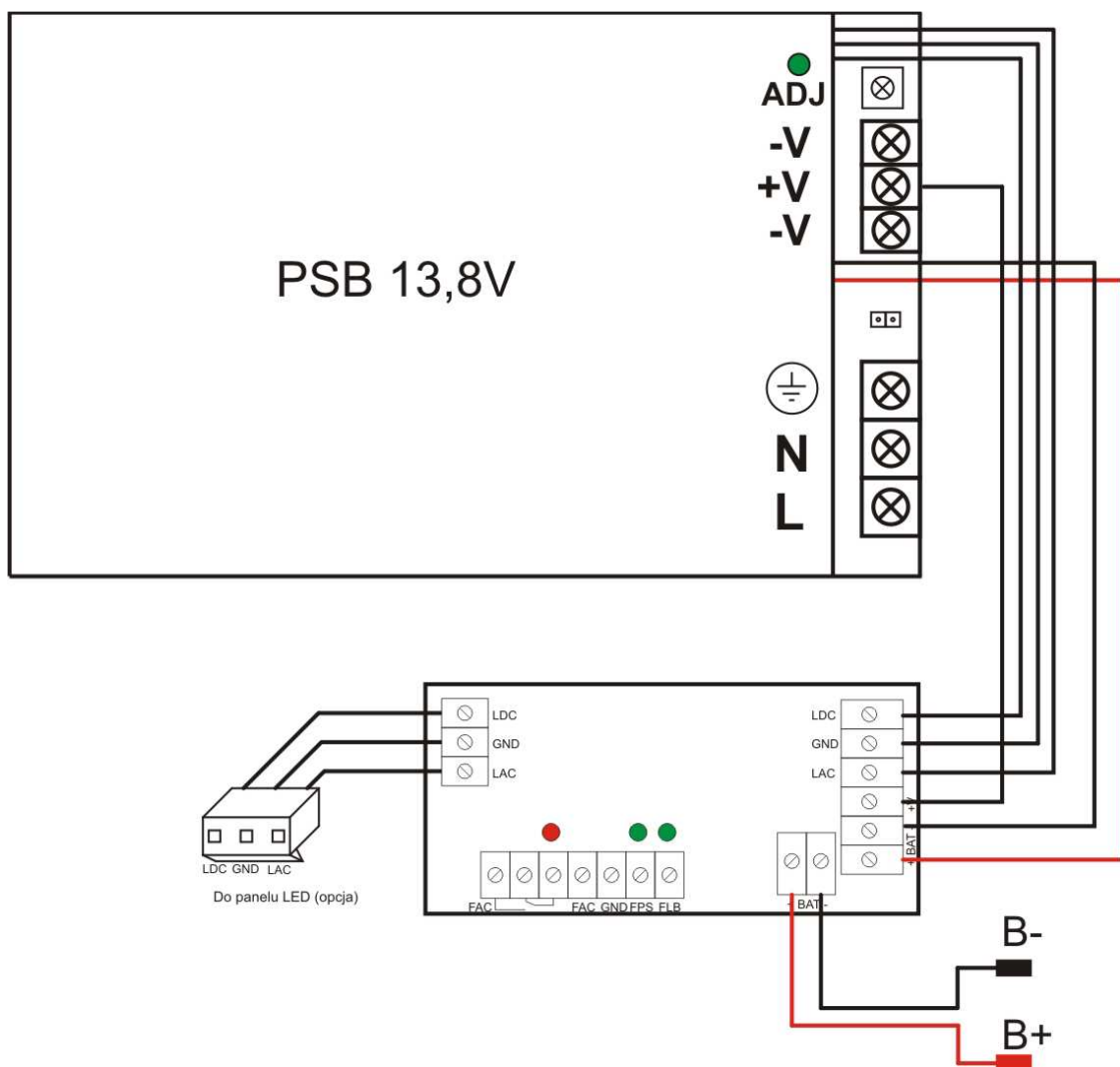
Rys.2 Schemat podłączenia modułu do zasilacza PSB.
