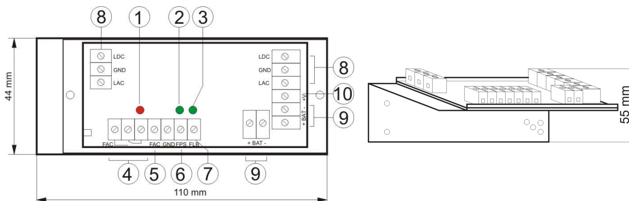
Rys.1 Widok modułu.
