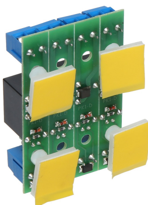
Rys. 2 Montaż za pomocą podstawek montażowych samoprzylepnych (PK4-XX-ZN).
