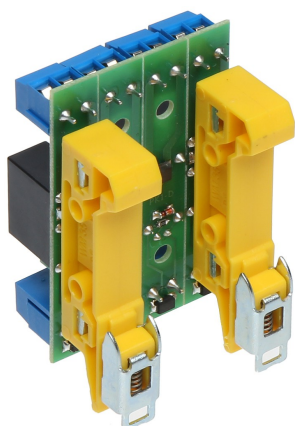
Rys. 1 Montaż na szynie DIN za pomocą podstawek montażowych WM-35 i dystansów 3mm (PK4-XX-ZD).
