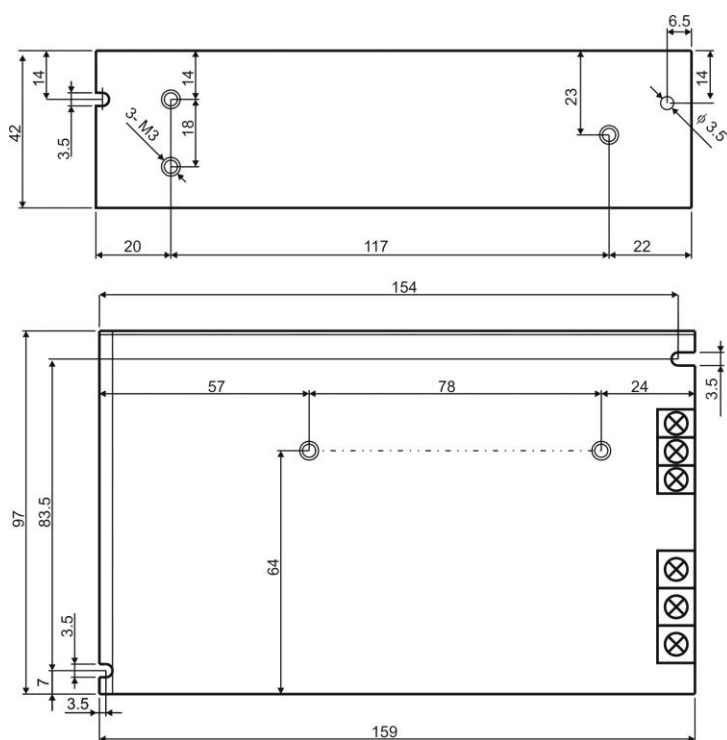
Rysunek 2. Widok mechaniczny zasilacza
