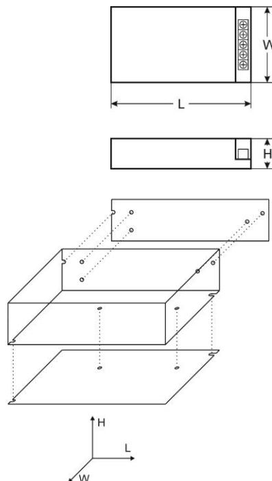
Rysunek 2. Widok mechaniczny zasilacza
