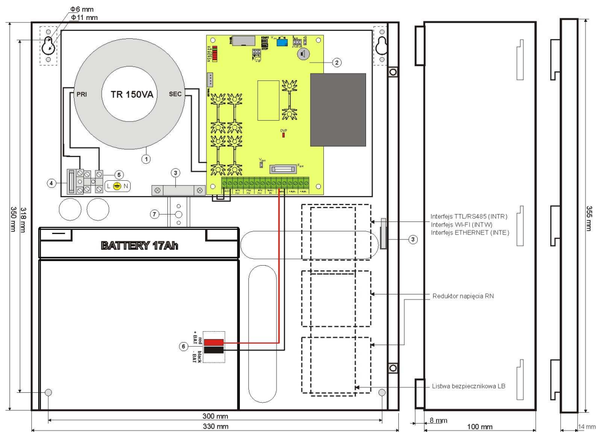
Rys.3. Widok zasilacza.
