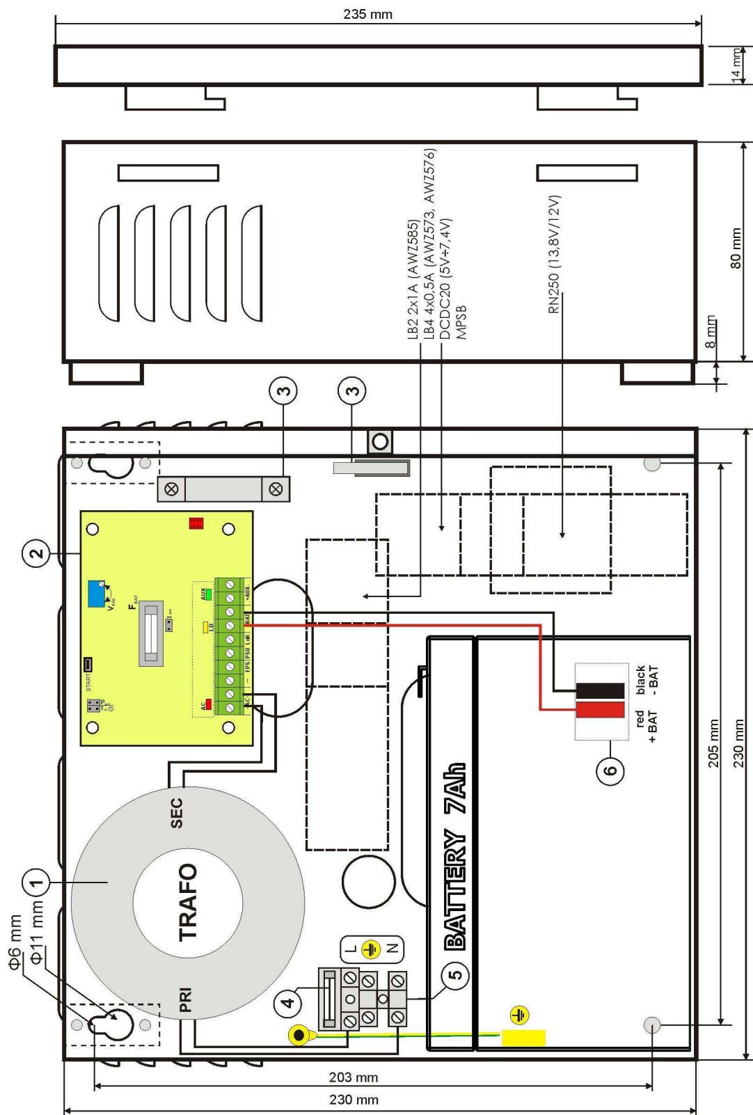
Rys.3. Widok zasilacza.
