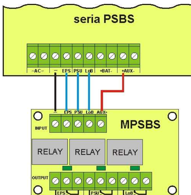
Rys. 5. Schemat podłączenia modułu MPSBS.
