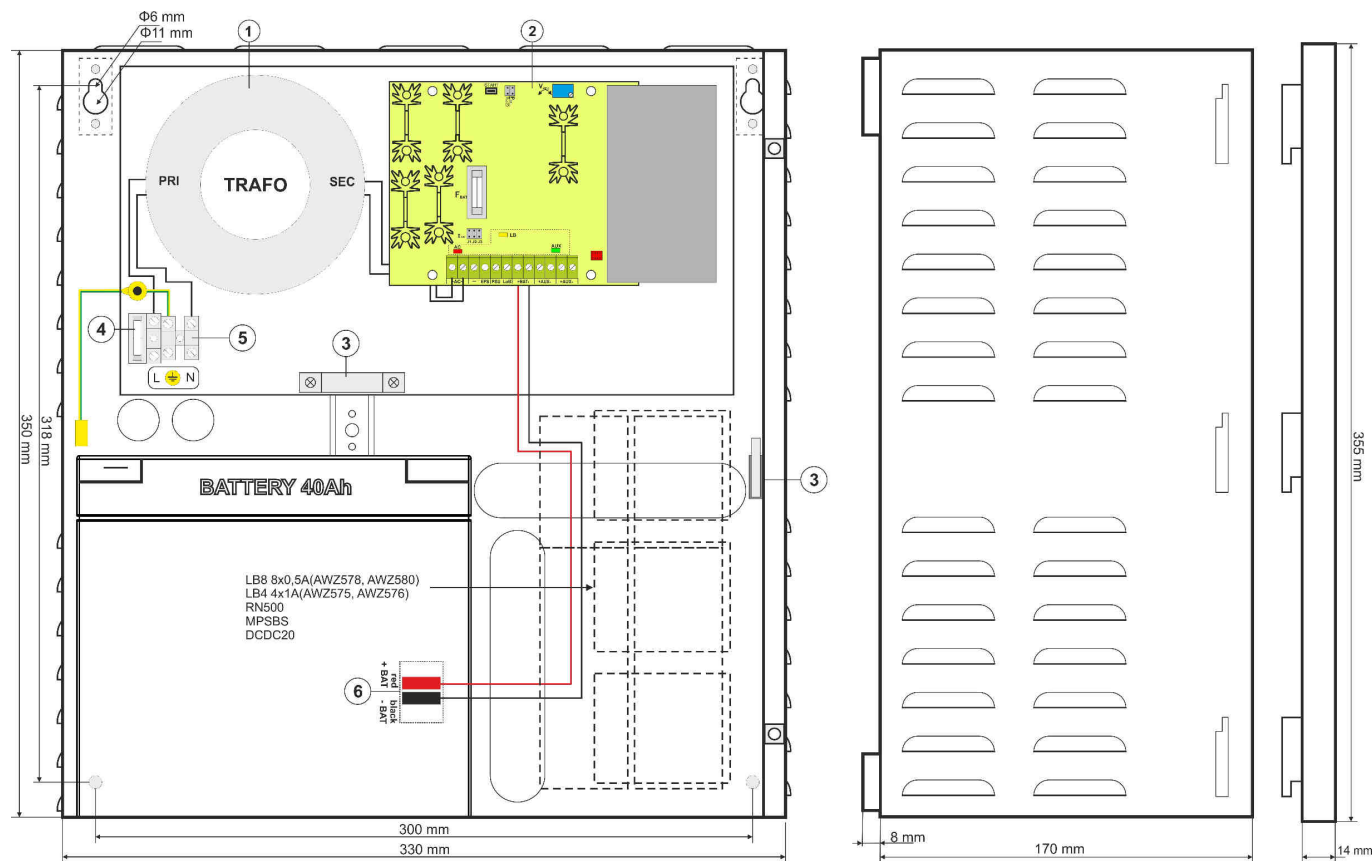
Rys.3. Widok zasilacza.
