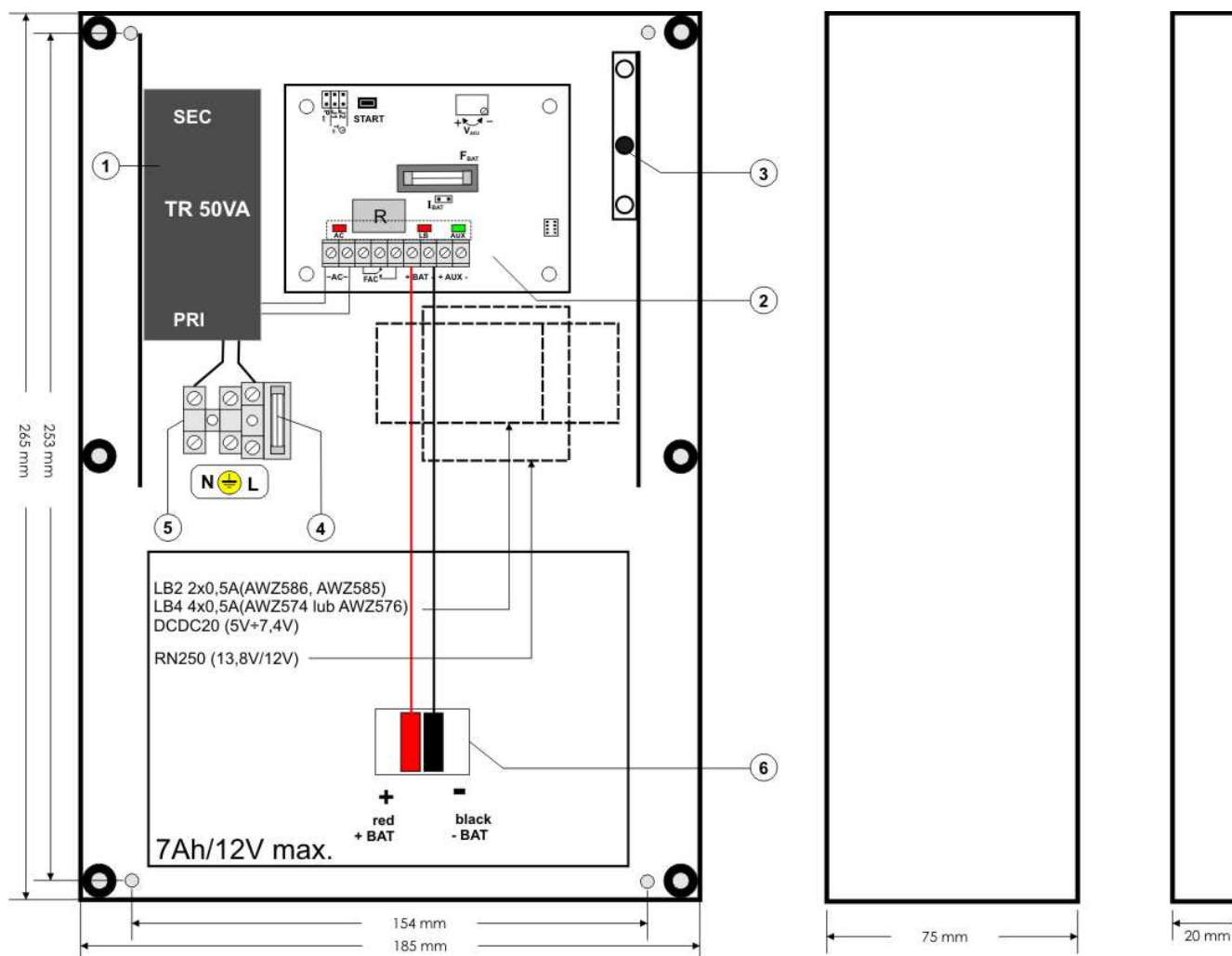
Rys.3. Widok zasilacza.
