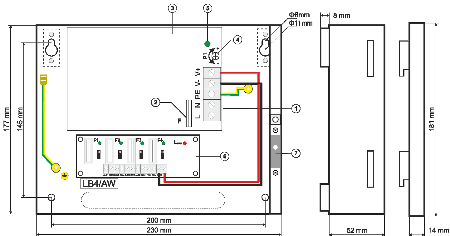
Rys.3. Widok zasilacza.
