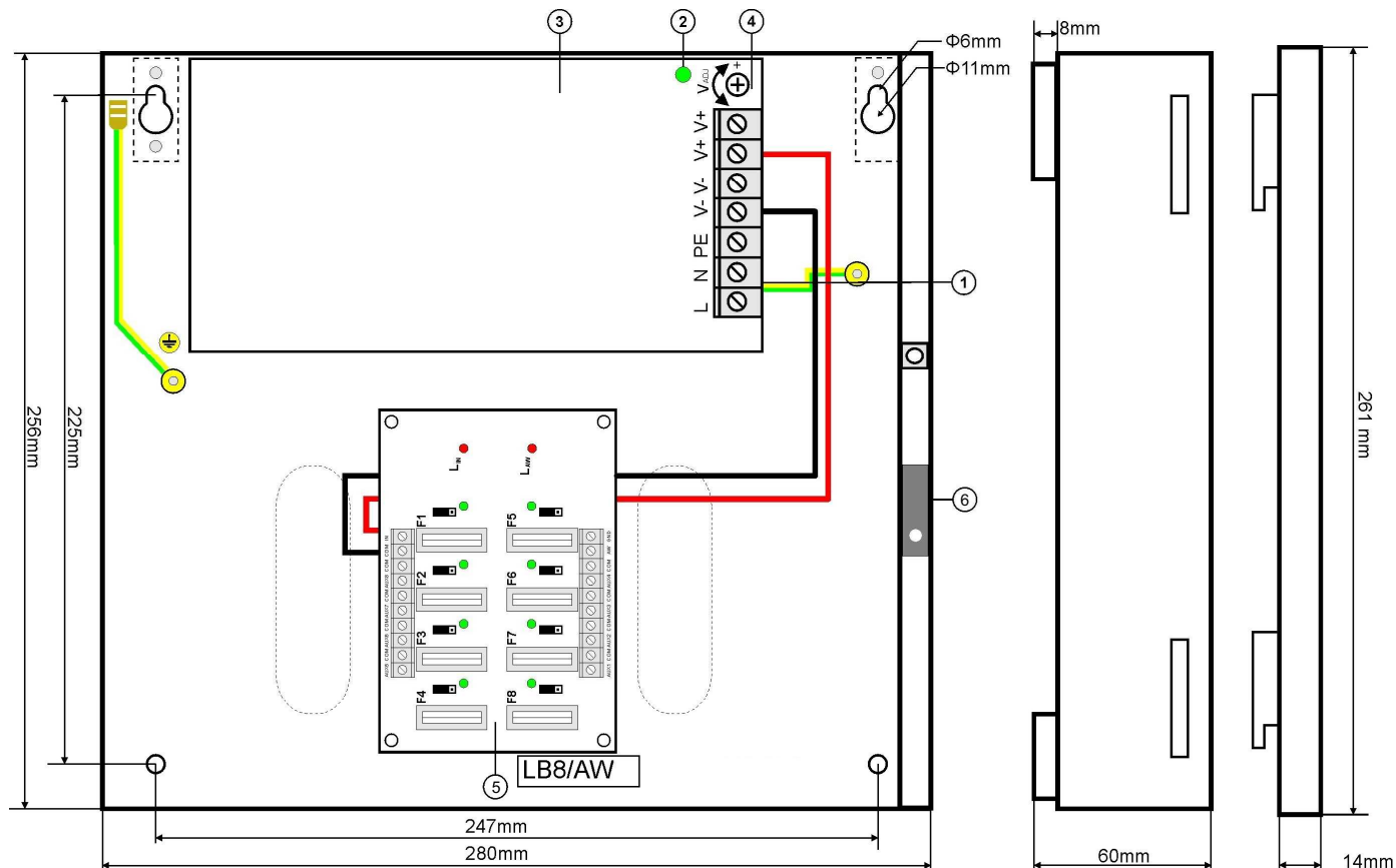
Rys.3. Widok zasilacza.
