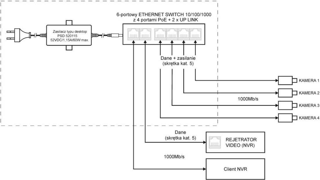
Rys 1. Schemat blokowy.
