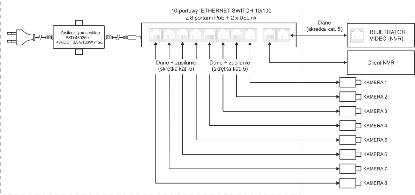
Rys. 1. Schemat blokowy.
