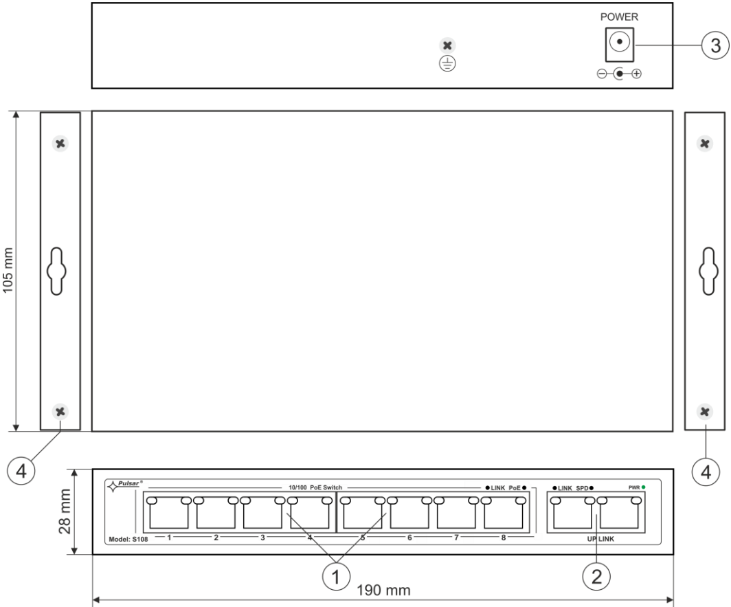
Rys. 2. Widok switch'a.
