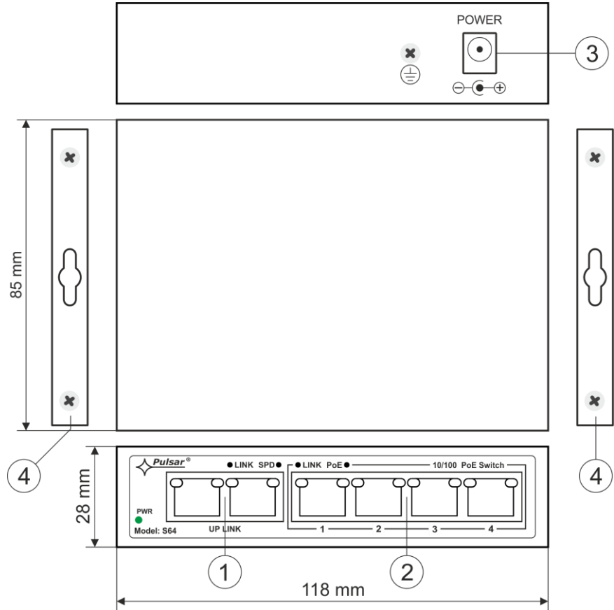
Rys. 2. Widok switch'a.
