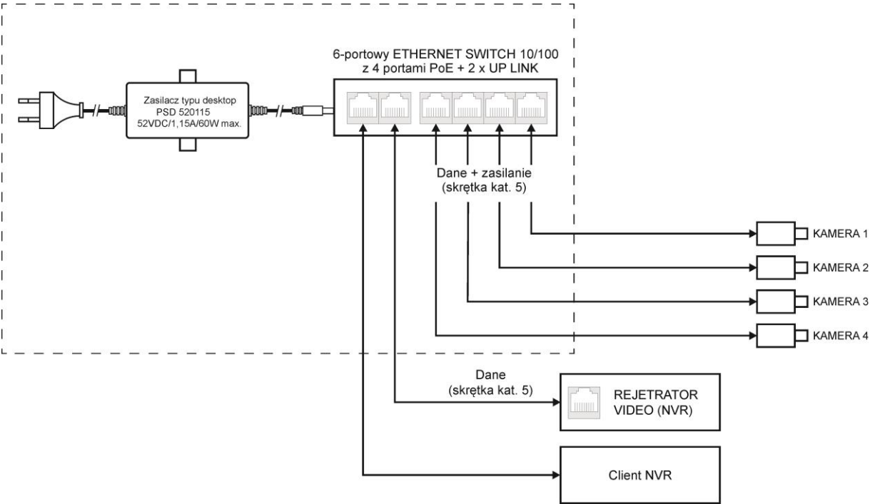
Rys. 1. Schemat blokowy.
