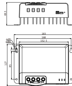
Model : MC2450N10 ; Outline dimensions : 183*127*69.5mm ; Mounting dimensions : 168*85mm ; Fixed holes dia : \Phi 5mm ; Wire specifications : 20-6AWG.
