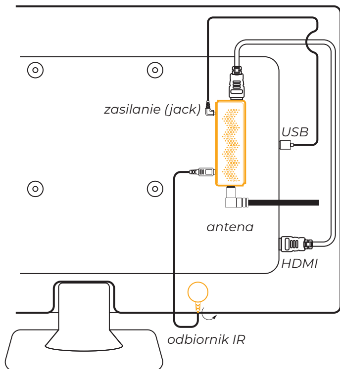
Schemat podłączenia odbiornika do TV
