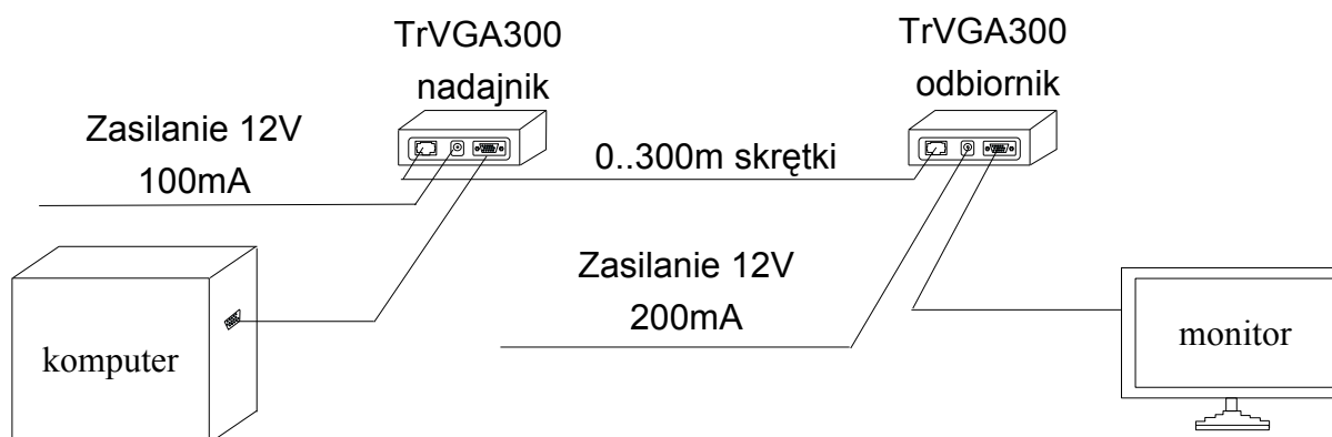
Rys. 1 Schemat połączeniowy nadajnika i odbiornika TrVGA300
