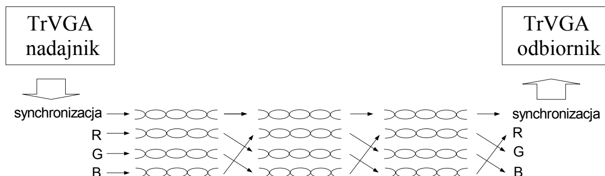
Rys. 2 Schemat działania przeplotu, kompensującego różnicę długości poszczególnych par skrętki
